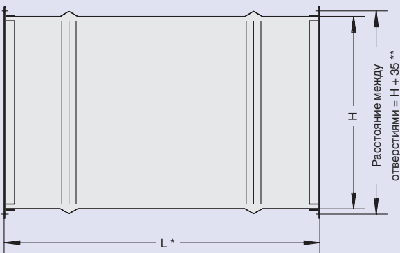
Пластиночтатый шумоглушитель НСВК...
