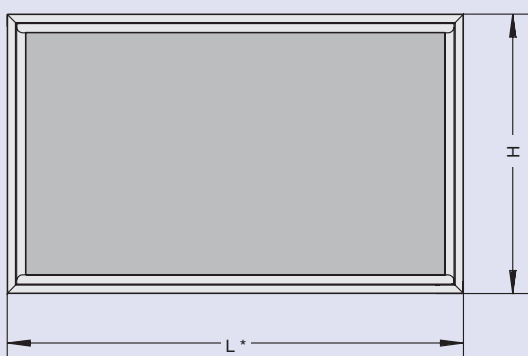
Шумопоглощающая пластина НСВКР...
