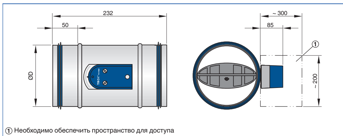
CAV регулятор Вариант PBMHC/.../E0*, с сервоприводом (потенциометры)
