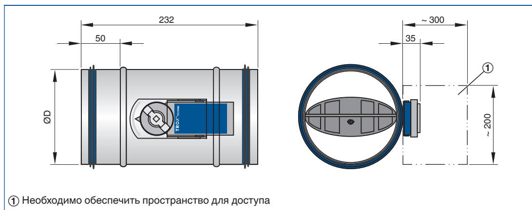
CAV регулятор Вариант PBMHC/.../M0*, с сервоприводом (механические ограничители)
